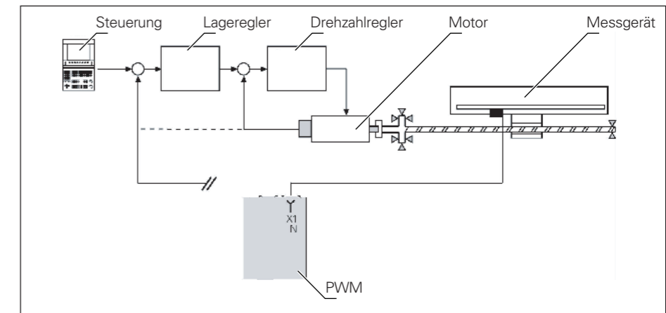
Messgeräte-Diagnose
